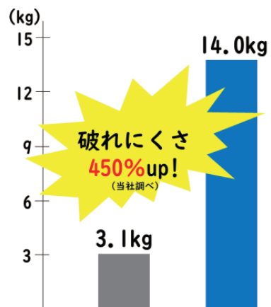
エアパンク試験
